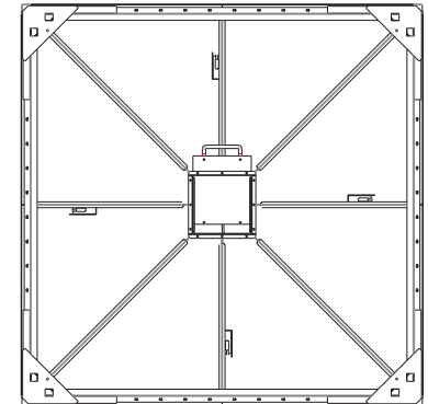
Abb: Silo Draufsicht, Schieber 300x300 mm
