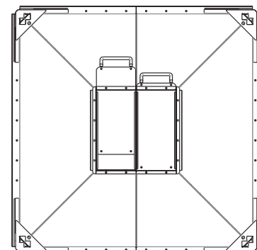
Abb: Silo Draufsicht, geteilter Schieber 500x500 mm
